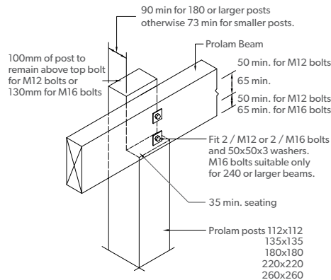
BEAM FIXING (D)
